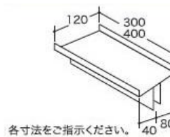
道具受皿
