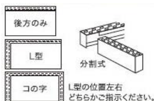
排気枠
